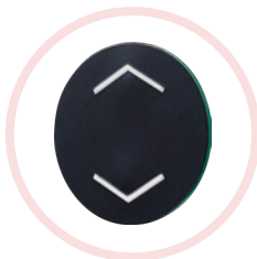
TFH13
