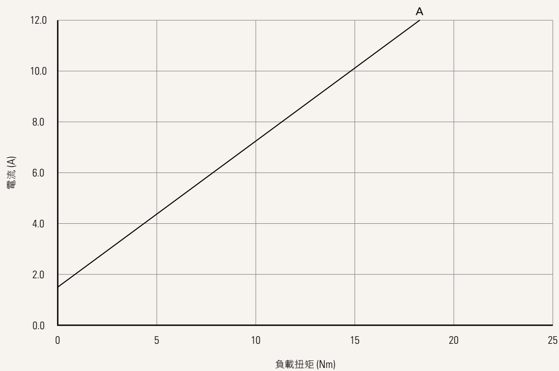
電流 vs. 負載扭矩
