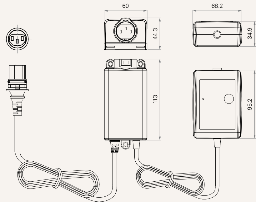
TEB2連接到控制盒之AC線
